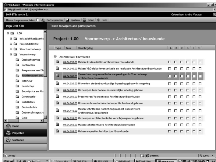
Figuur 8: Het navigeren door de STB met behulp van computerapplicatie dnrstb.nl (Screenshot van het programma dnrstb.nl testversie 2.1 met STB versie 2009).
